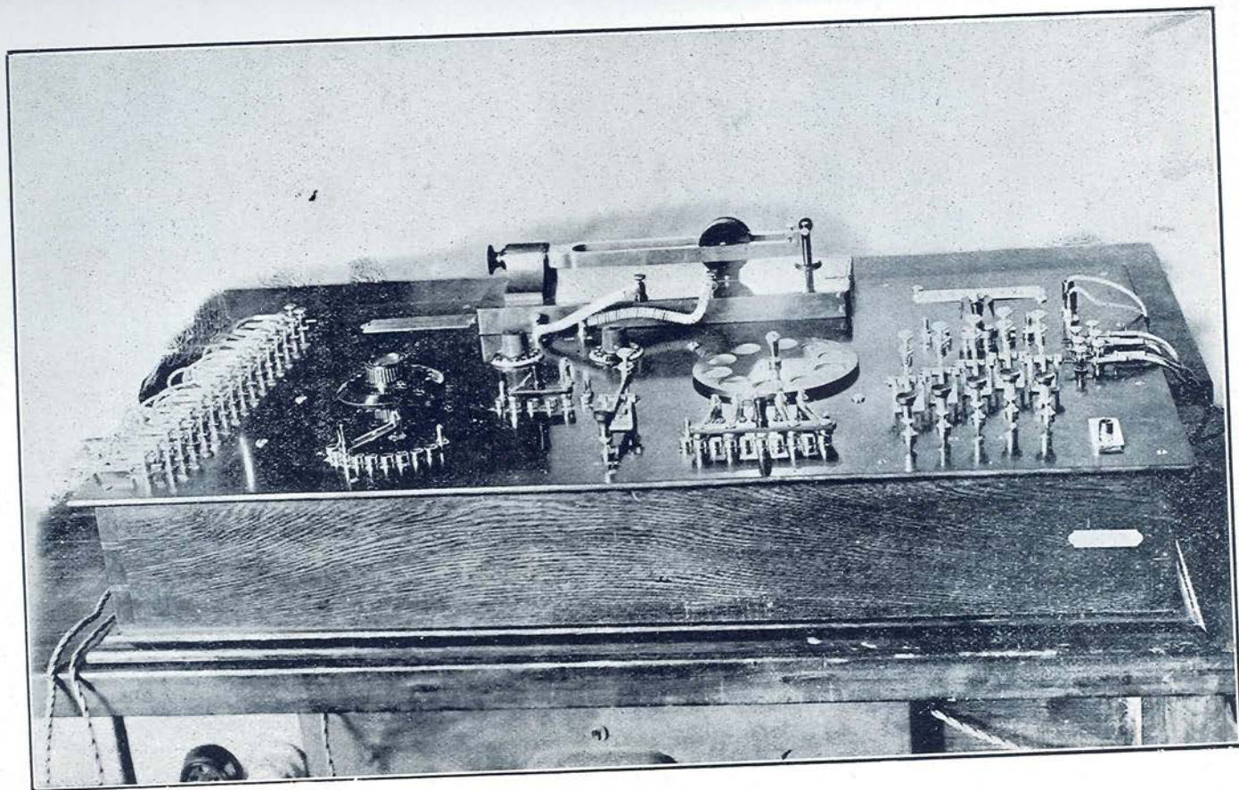
Registrador de los Profs. Mó y Alberti--Tablero del Operador
