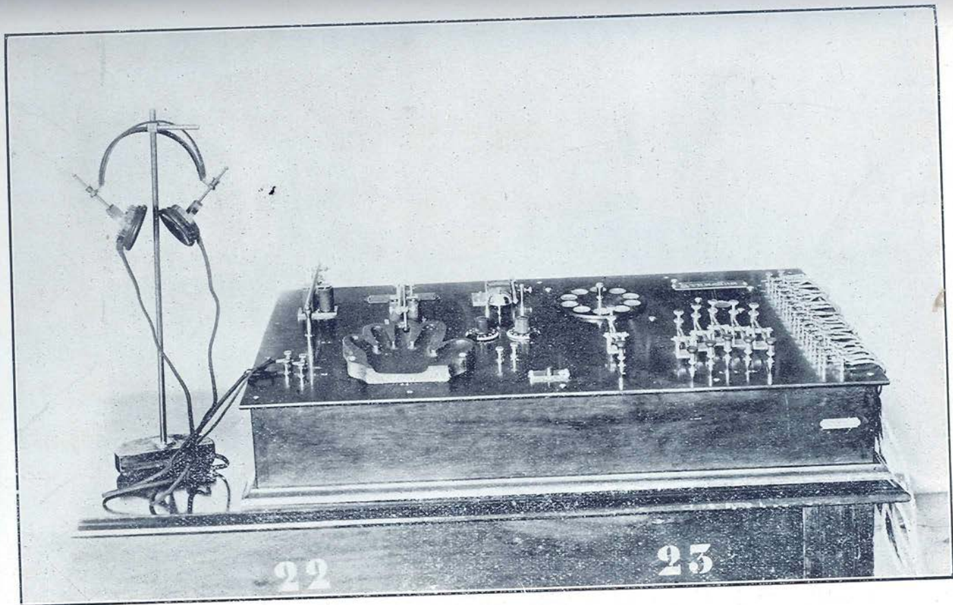
Registrador mental de los Profs. Mó y Alberti—Tablero del Sujeto
