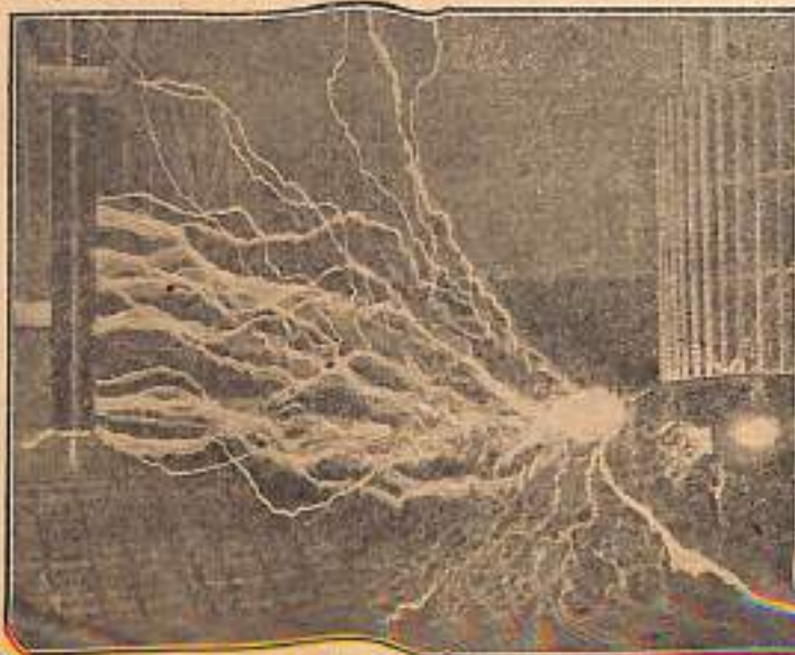
Descargas que sirven para crear en la tierra conexiones eléctricas que pueden llegar a los planetas.
