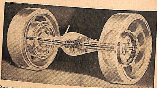
Puente trasero del poderoso camión White. AB, primera reducción; C, eje palier; DEF, segunda reducción; G, tambor de freno; H, guardapolvo.
