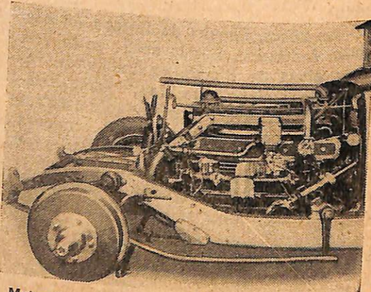
Motor Continental aplicado en el coche Aerotype.
