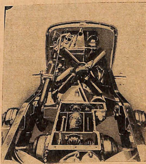
Detalles de la propulsión delantera del motor Continental de 8 cilindros aplicado en el coche Aerotype 1930.
