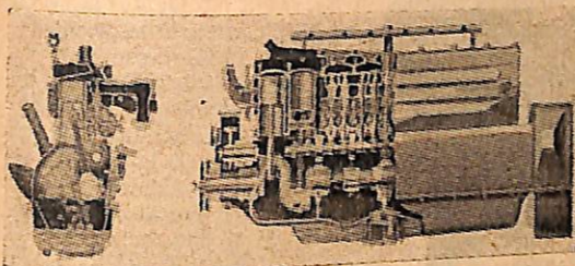
El motor 8 cilindros del coche Gardner visto de frente y de costado. Este motor ha sido preparado en el país y con él Cayetano D'Amico ganó la carrera de las 500 millas de Rafaela.
